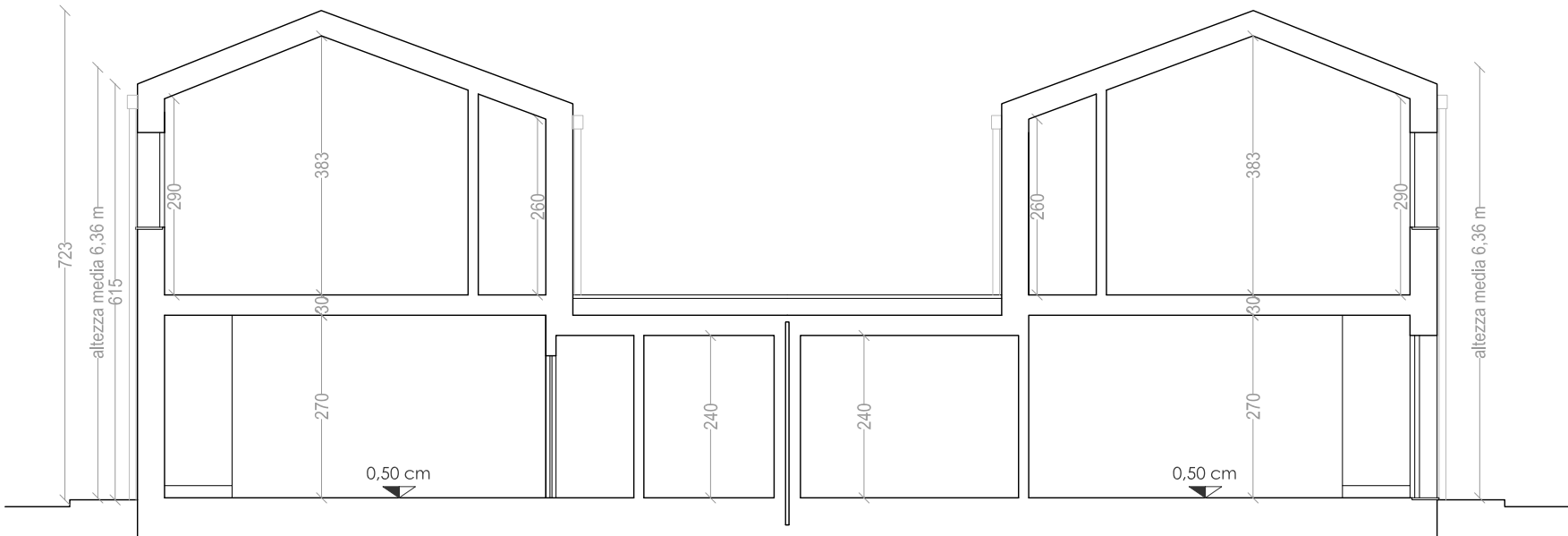
SEZIONE AA
