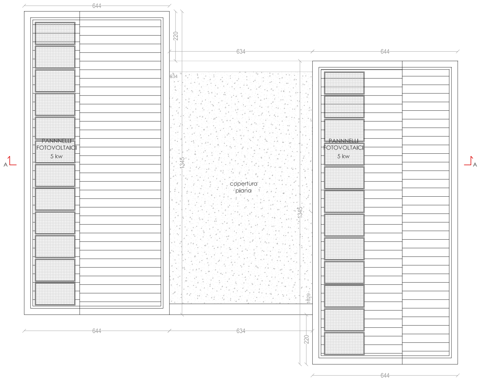
COPERTURA
